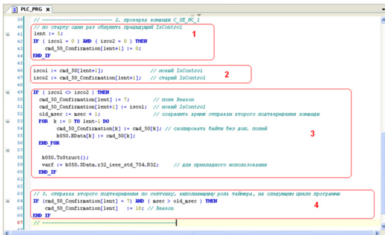
Рисунок 25 – Модуль ASDU. PLC_PRG область отображения пользовательской задачи. Команда cmd_50
