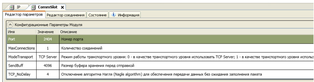
Рисунок 28 – Конфигурационные параметры CommSlot . Закладка Редактор параметров
