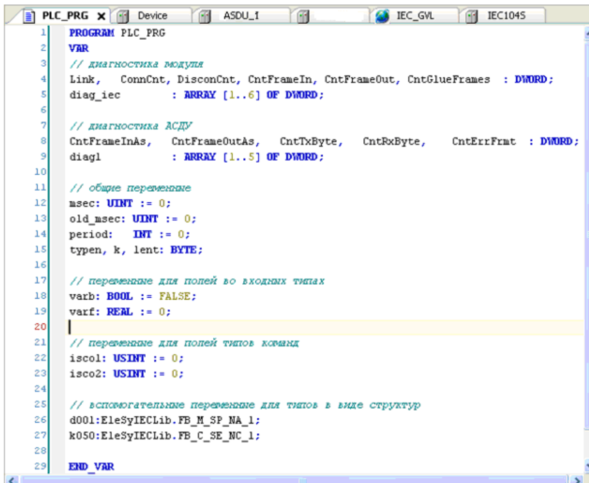
Рисунок 23 – Модуль ASDU. PLC_PRG область отображения процедуры объявления переменных проекта
