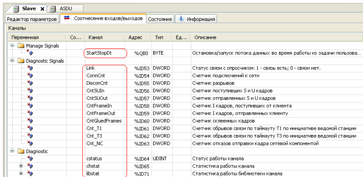
Рисунок 34 – Модуль Slave . Закладка Соотнесение входов/выходов
