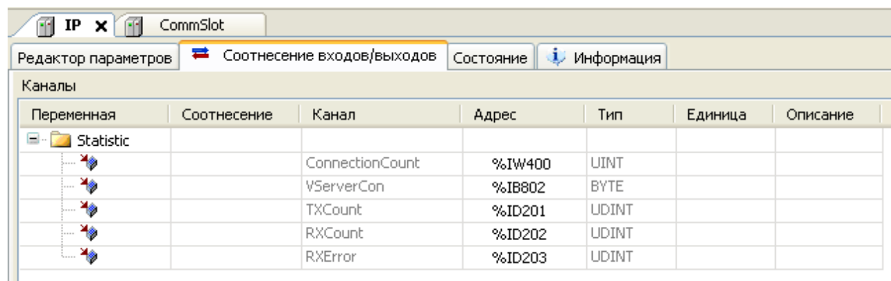
Рисунок 27 – Модуль IP. Закладка Соотнесение входов/выходов
