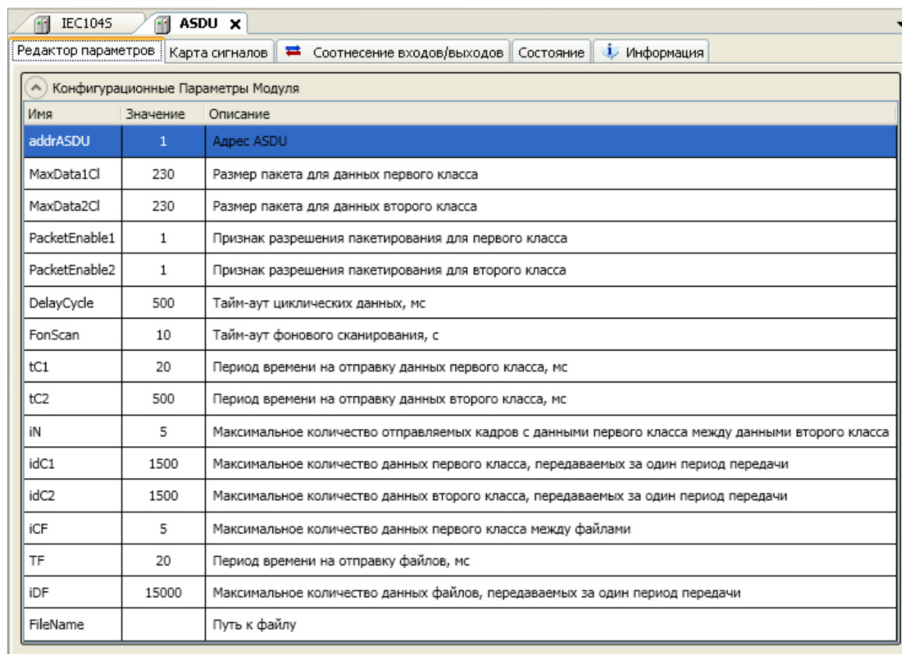
Рисунок 8 – Модуль ASDU. Закладка Редактор параметров
