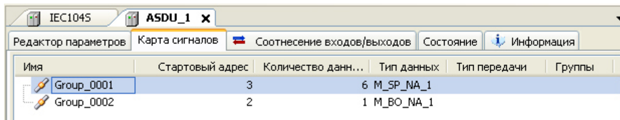
Рисунок 12 – Модуль ASDU. Закладка Карта сигналов
