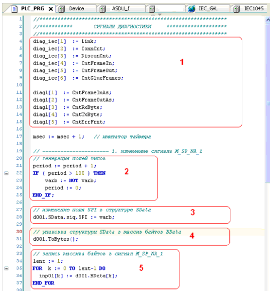
Рисунок 24 – Модуль ASDU. PLC_PRG область отображения пользовательской задачи. Сигнал inp01
