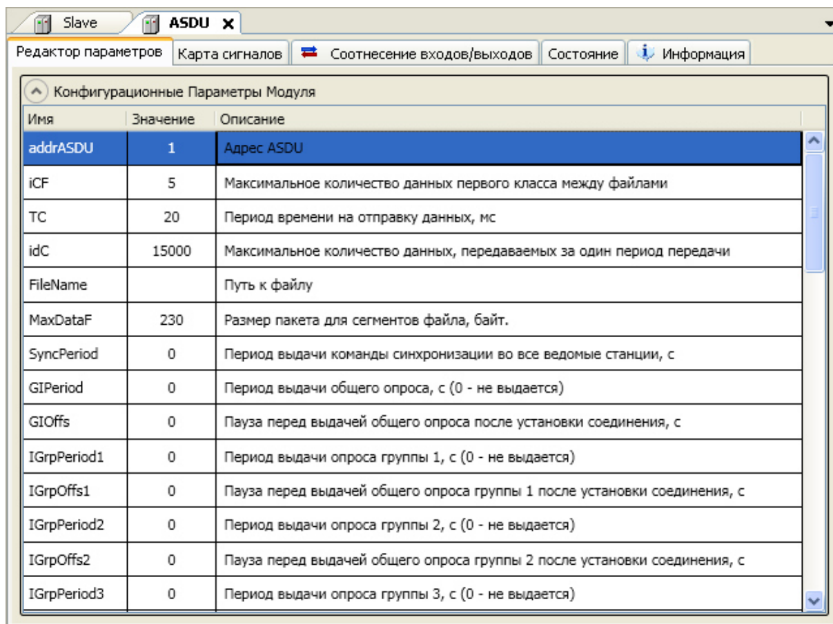
Рисунок 35 – Модуль ASDU. Закладка Редактор параметров
