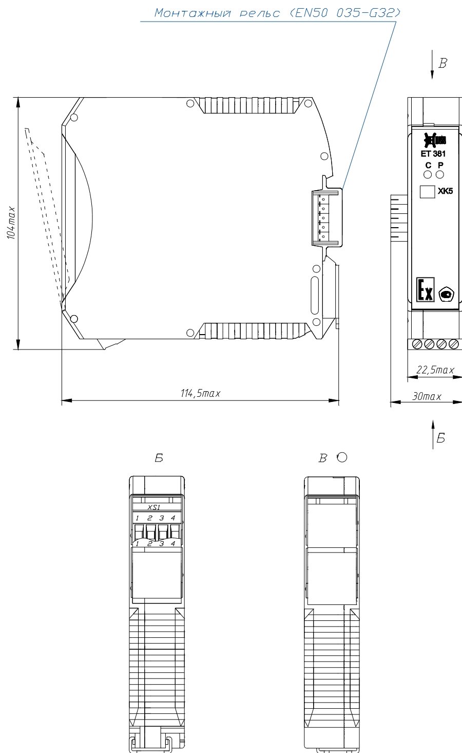
Рисунок А.1 – Габаритный чертеж преобразователя ET 381
