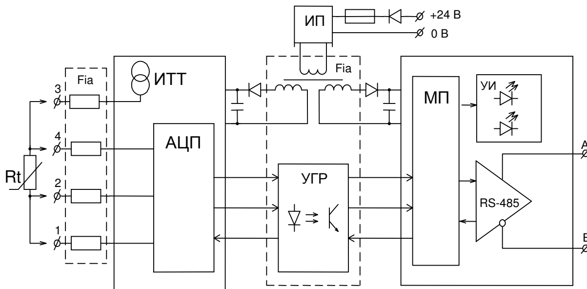
Рисунок 1 – Структурная схема преобразователя ЕТ 381
