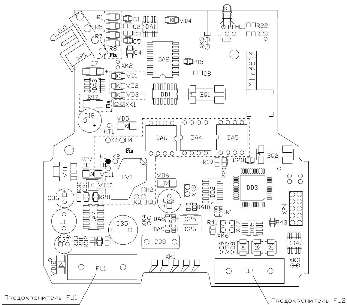
Рисунок Б.1 – Схема размещения элементов на плате преобразователя ET 381
