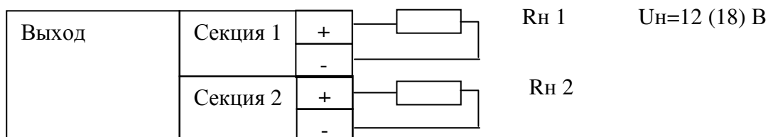
Рисунок 3 – Схемы включения выхода
