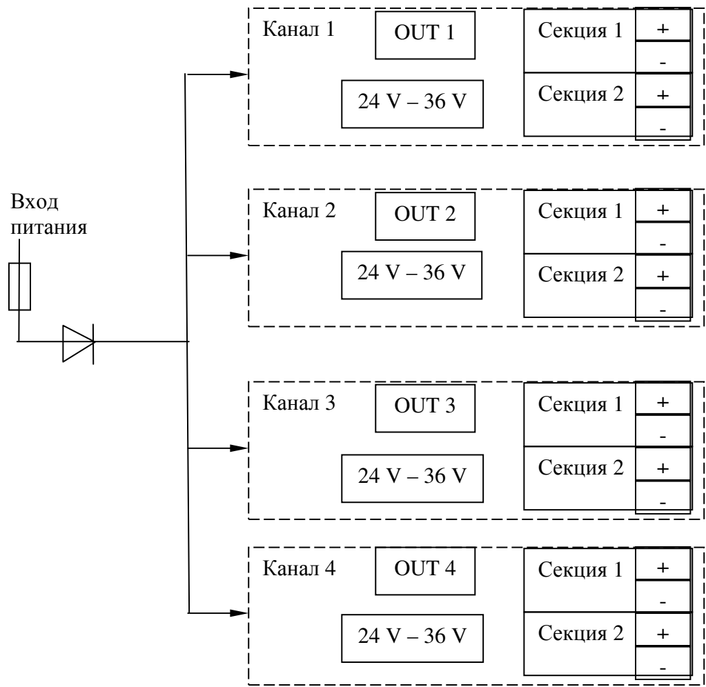
Рисунок 1 – Структурная схема модуля
